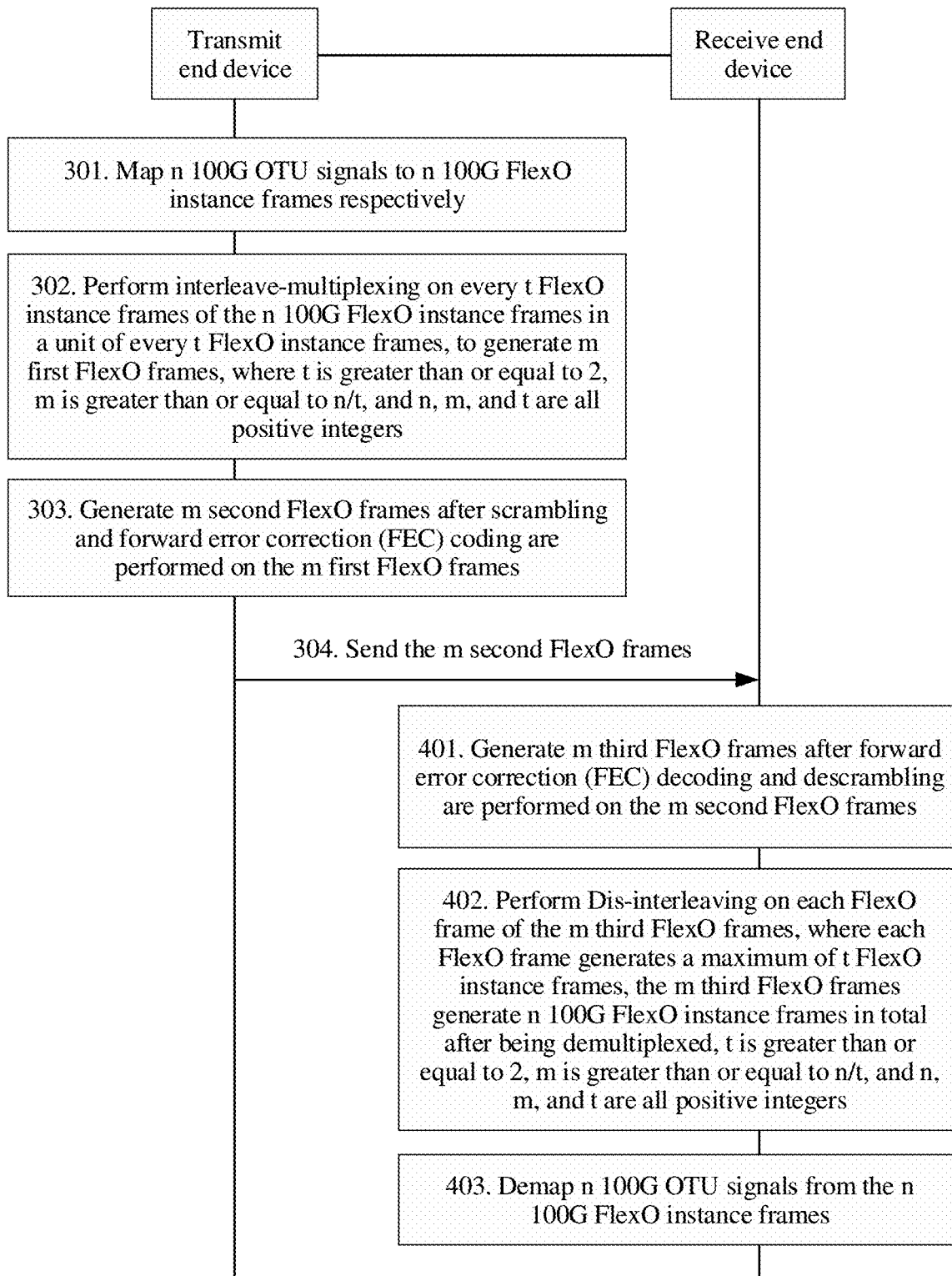
FIG. 3B
