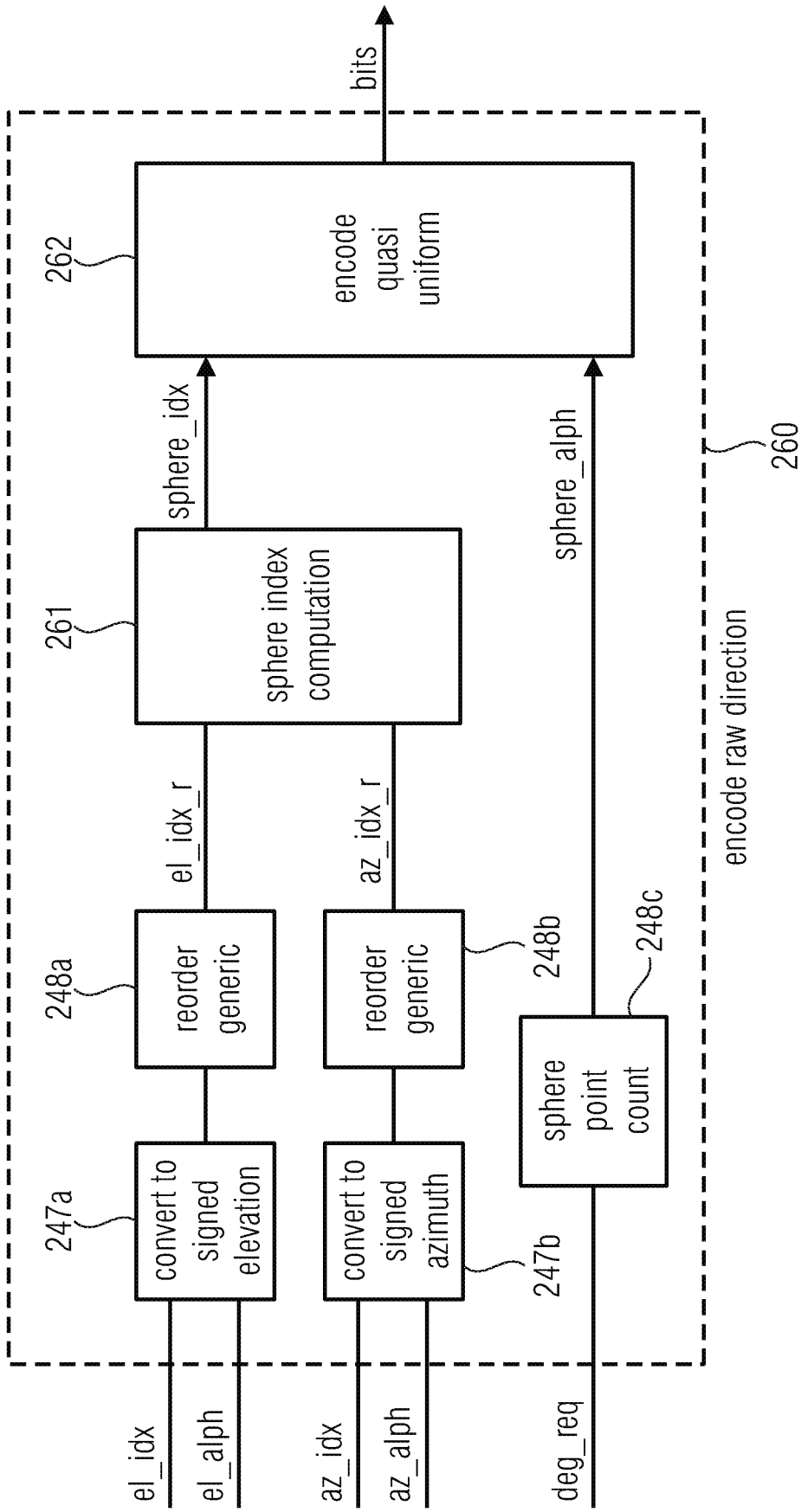
Fig. 6c Encoder
