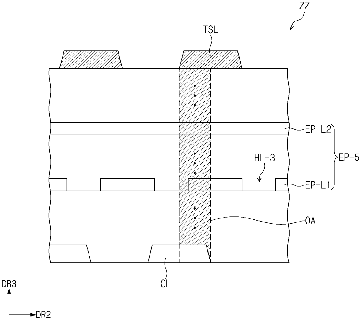
FIG. 11B
