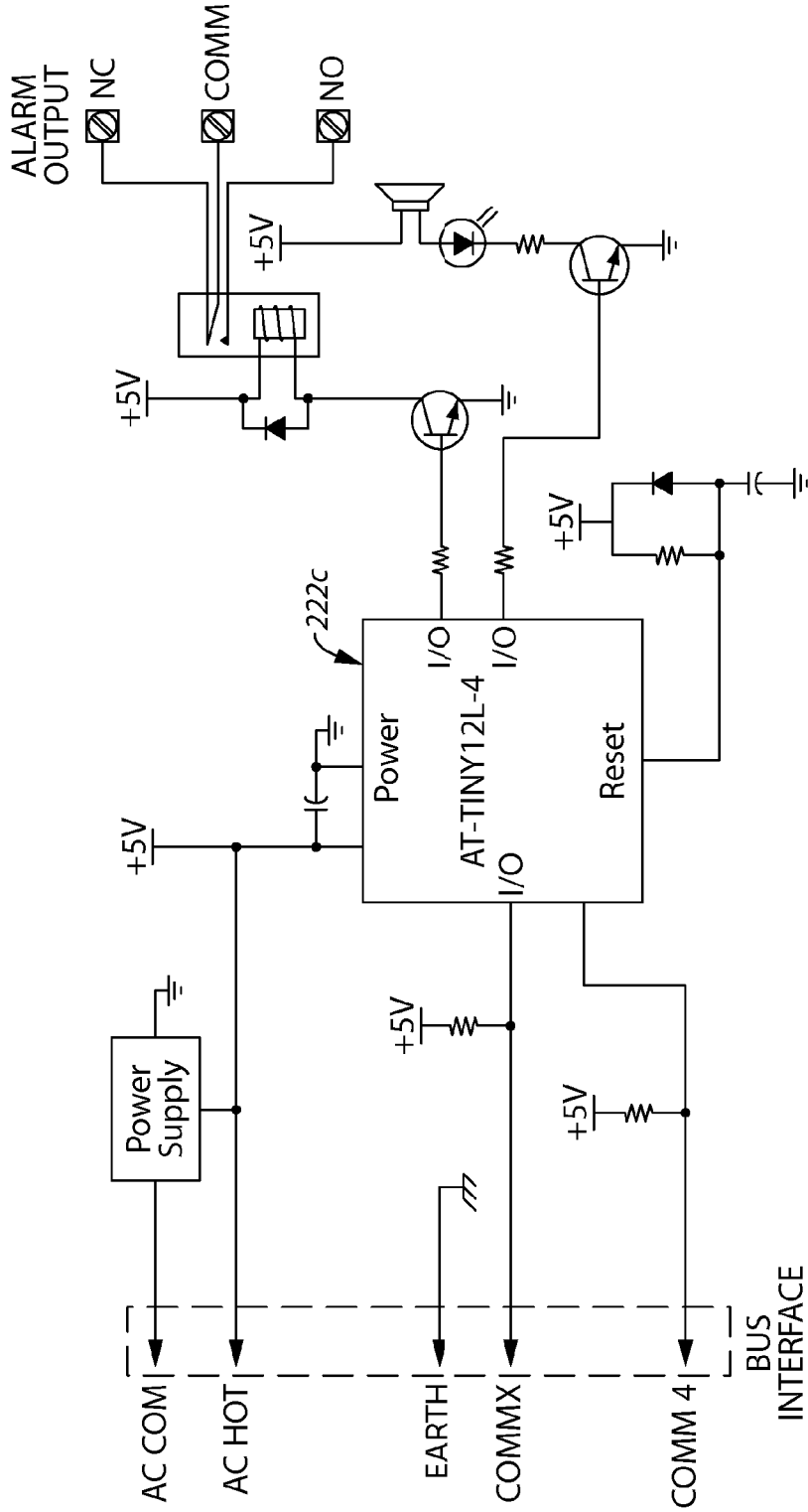
SMART MODULE 226
