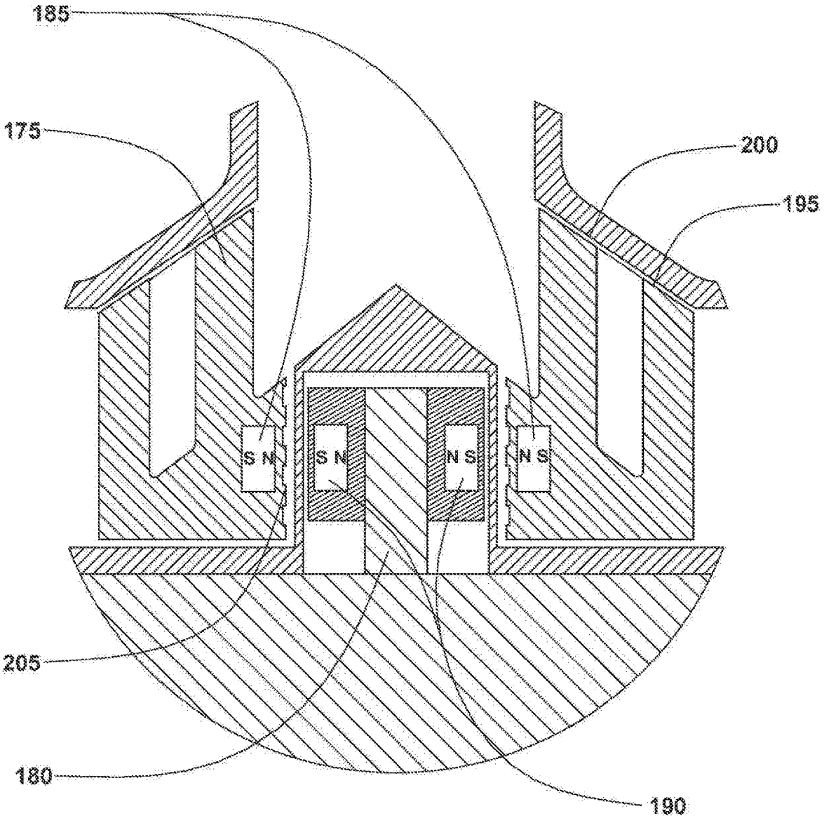
FIG. 17 (DETAIL E)
