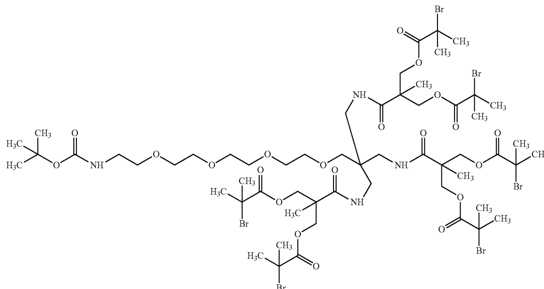
Compound F1
