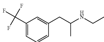
(RS)-N-ethyl-1-[3-(trifluoromethyl)phenyl]propan-2-amine
