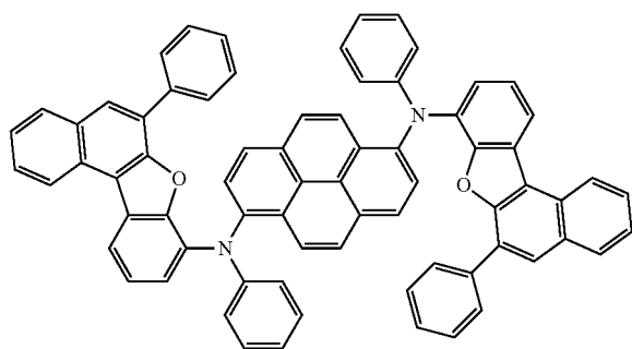
1,6BnfAPm-03
