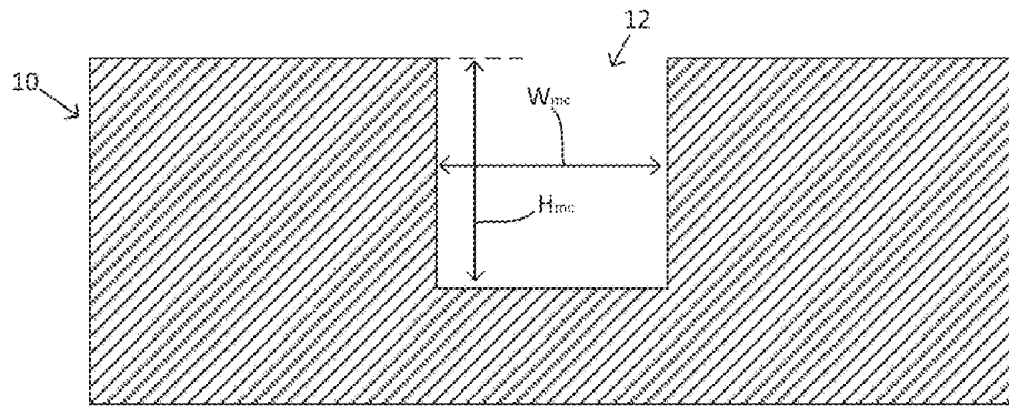
FIG. 6D
