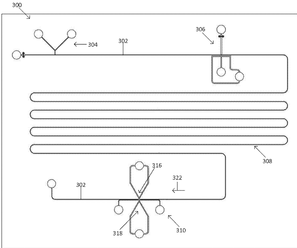
FIG. 16A
