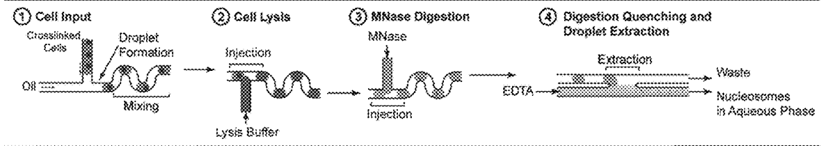
FIG. 1C
