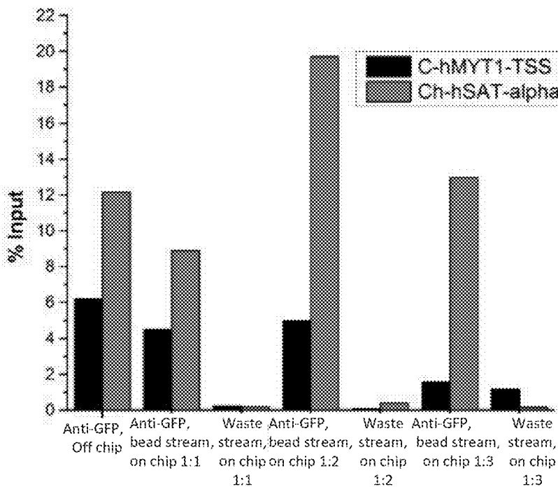
FIG. 5D
