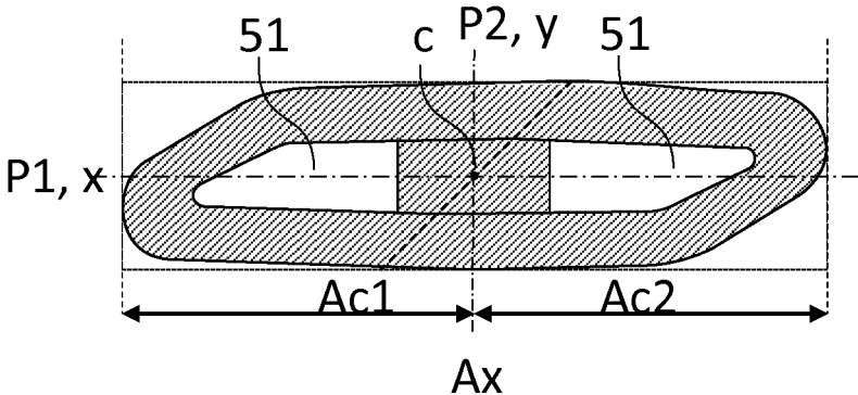
FIG.11 3-3
